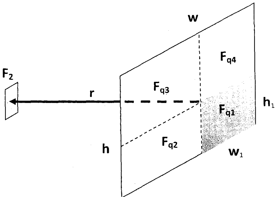
Рисунок А.3.2. Расположение излучающих поверхностей пламени Fq1-q4 и облучаемой поверхности материала соседнего объекта F2, где w1 и h1 - длина и ширина соответствующей части поверхности пламени.
